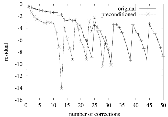
図 1: n = 128^2 での Jacobi 前処理の効果
